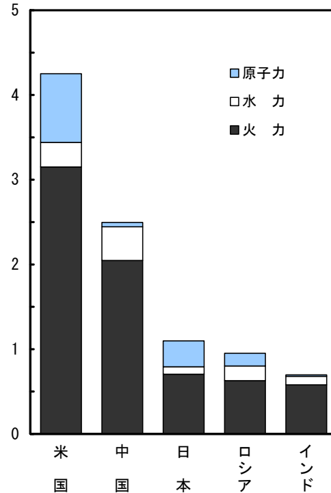
4 エネルギー別発電量 (2005年)
