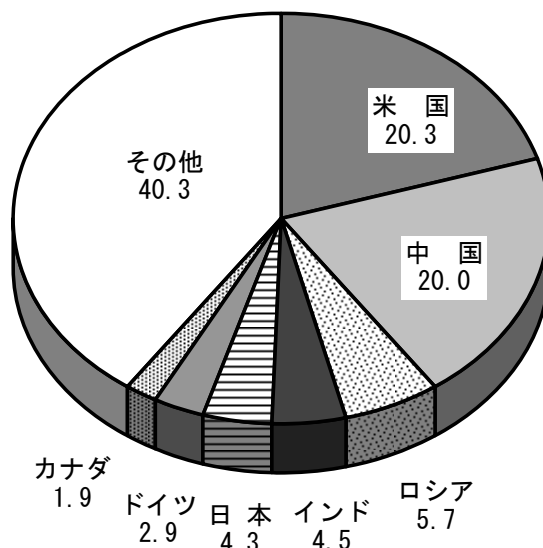
二酸化炭素排出量の各国構成比（2006年）
