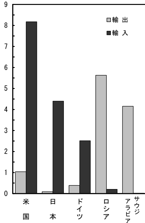
3 エネルギーの輸出入量 (2005年)
