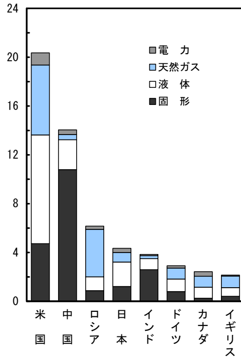
2 エネルギーの消費量 (2005年)
