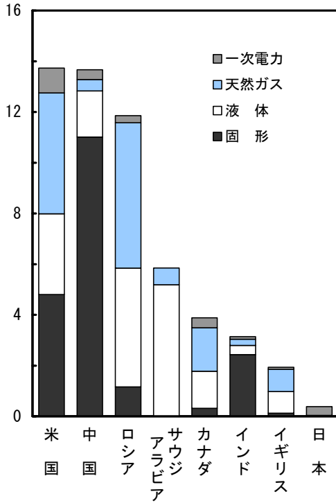
1 一次エネルギーの生産量 (2005年)
